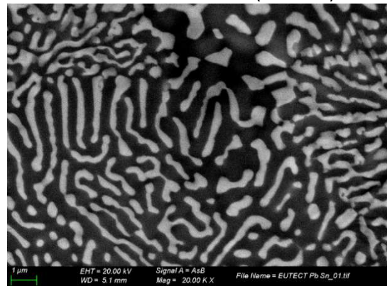
Material de soldadura (eutèctic)
